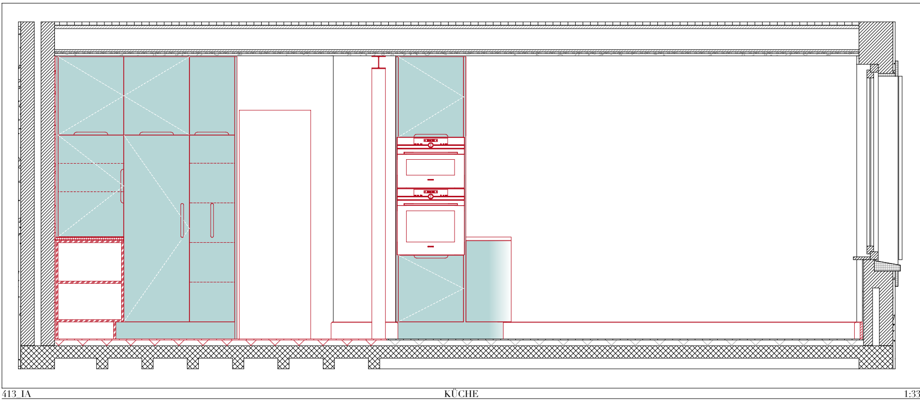
413 1A KÜCHE 1:33
