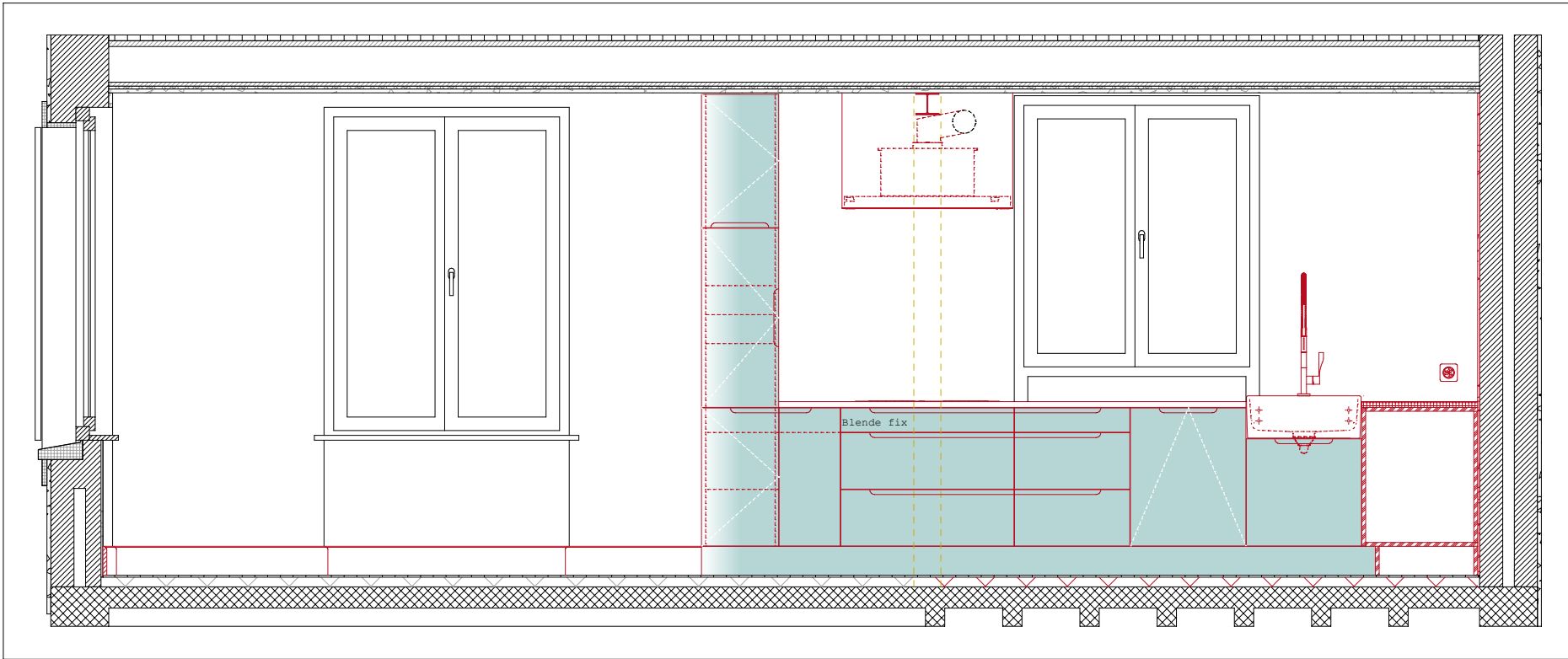
413 1A KÜCHE 1:33
