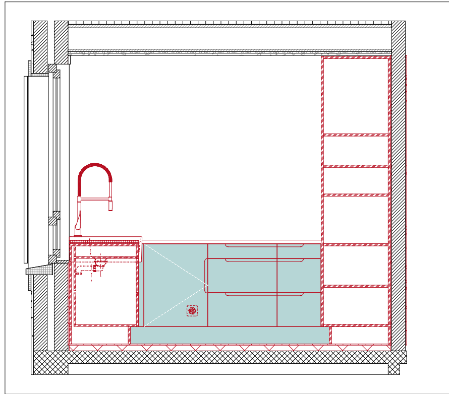
413 1A KÜCHE 1:33
