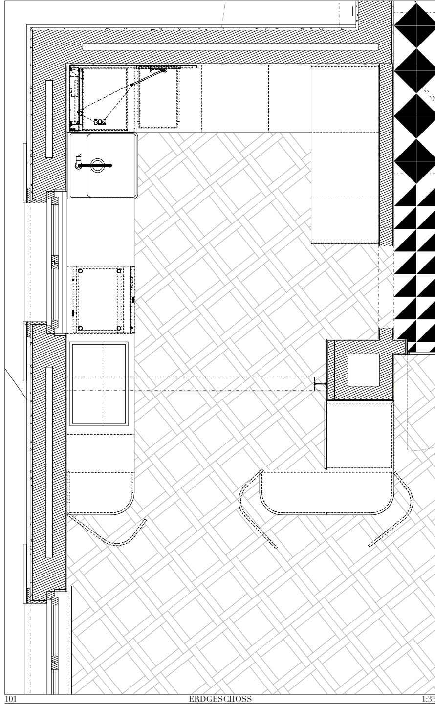
101 ERDGESCHOSS 1:33
