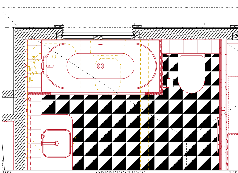
102 OBERGESCHOSS 1:33
