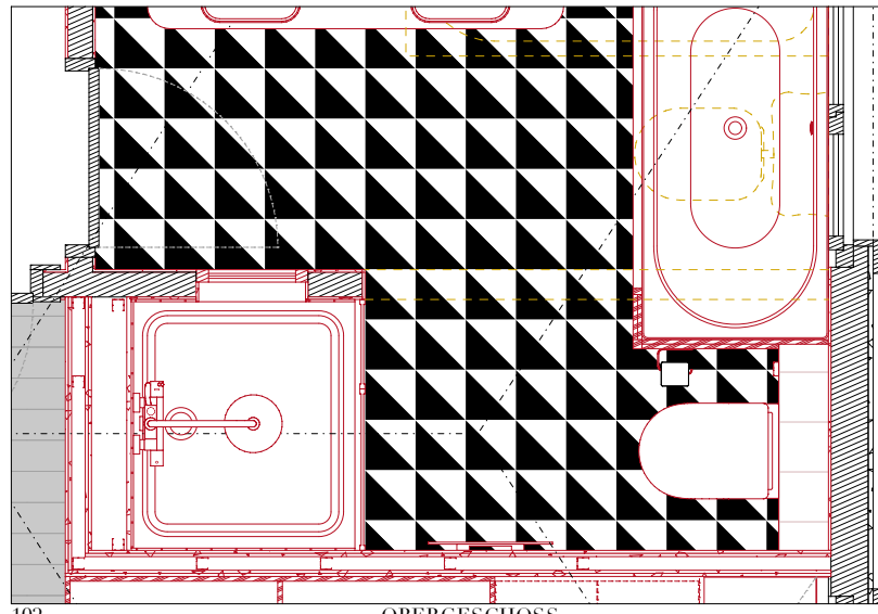
102 OBERGESCHOSS 1:33
