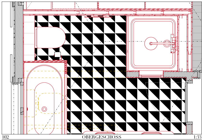
102 OBERGESCHOSS 1:33
