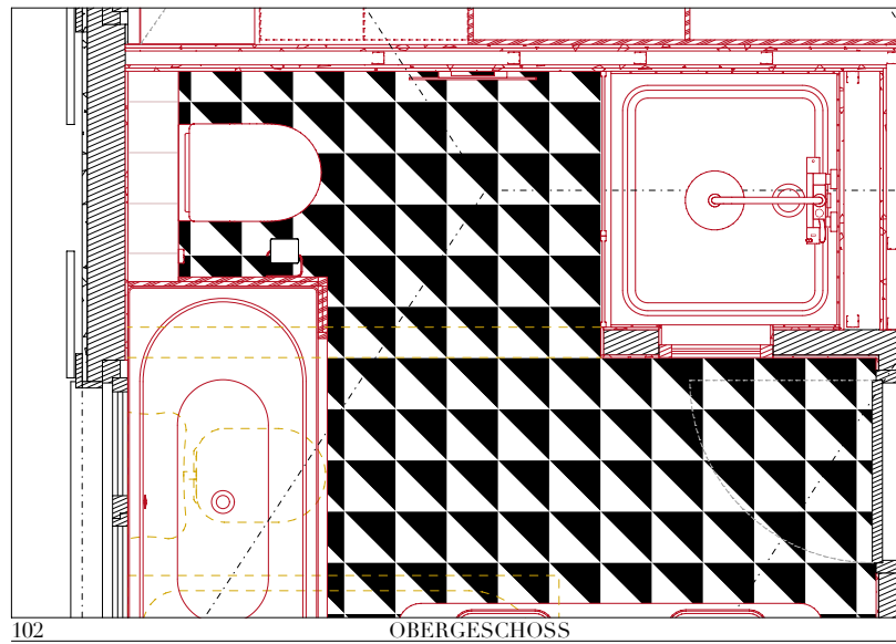
102 OBERGESCHOSS 1:33
