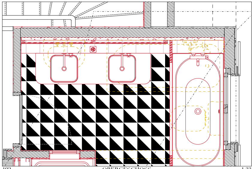
102 OBERGESCHOSS 1:33
