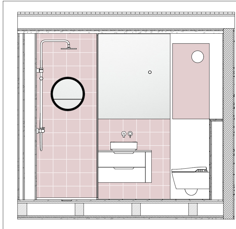
426 1A HAUPTBAD 1:33
