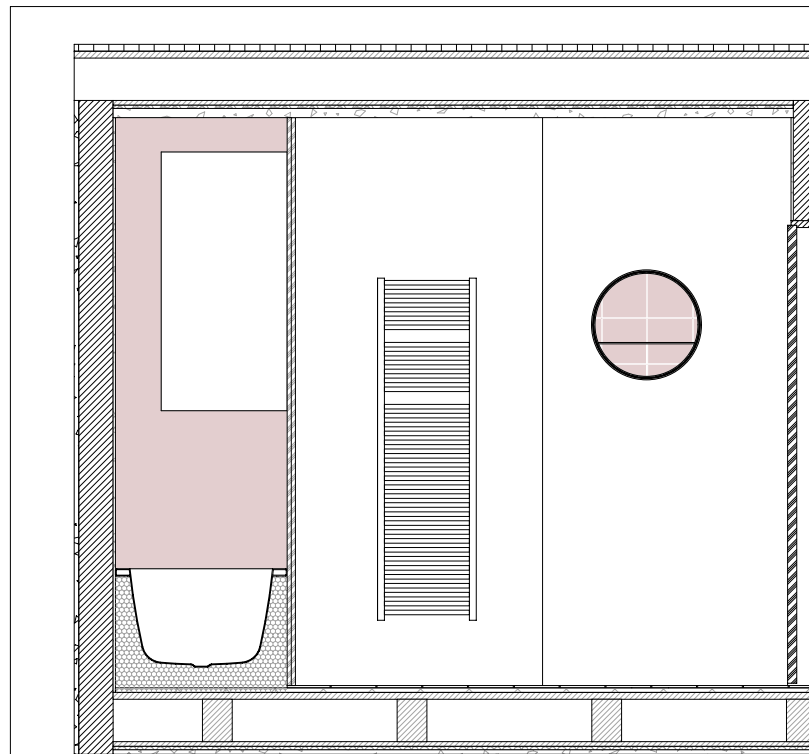
426 1A HAUPTBAD 1:33
