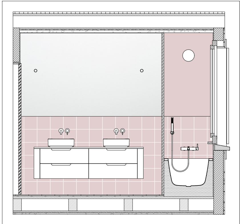
426 1A HAUPTBAD 1:33
