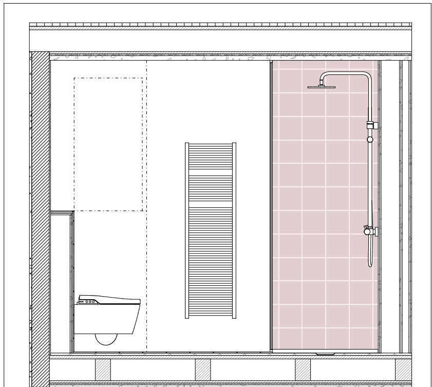
426 1A HAUPTBAD 1:33
